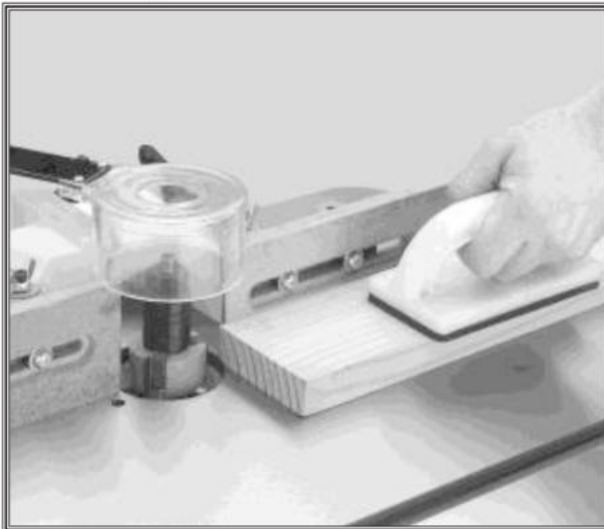
Figura 2. Utilice pisadores manuales Para detener la pieza al cortarla.
