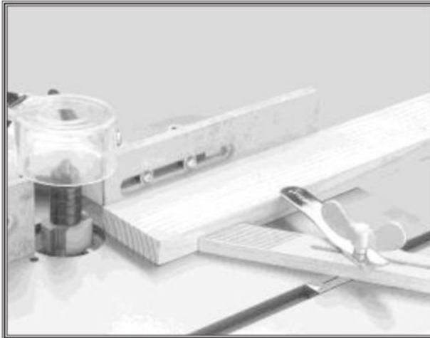
Figura 1. Utilice guías biceladas como protector.
